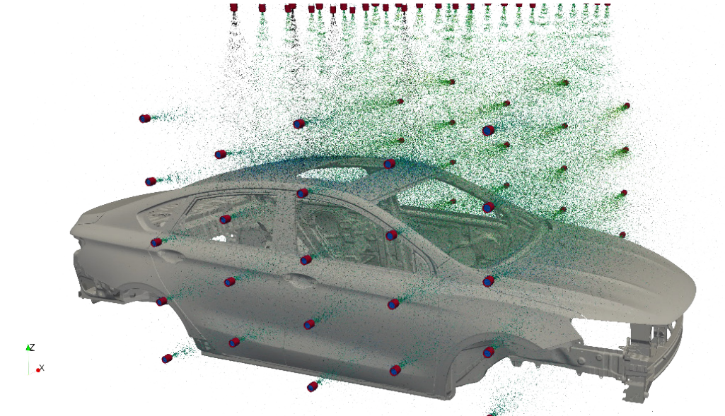
Spray & Rinse
